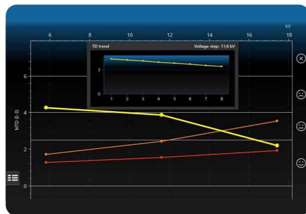
Znázornění měření ztrátového činitele v aplikaci BAUR verze 4 ↓
