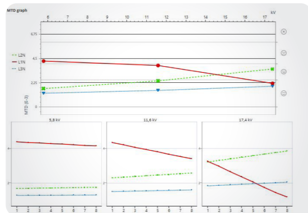
Znázornění měření ztrátového činitele ve zprávě ↑
