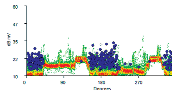
↑ Výsledek rychlé online zkoušky PD: Částečné výboje jsou znázorněny modře
