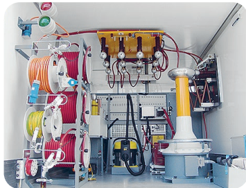
↑ Poloautomatický systém transcable, třífázový, 110 kV
